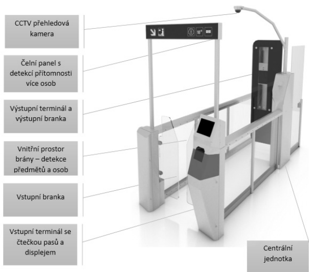
Obrázek č. 3: Základní popis eGate brány
